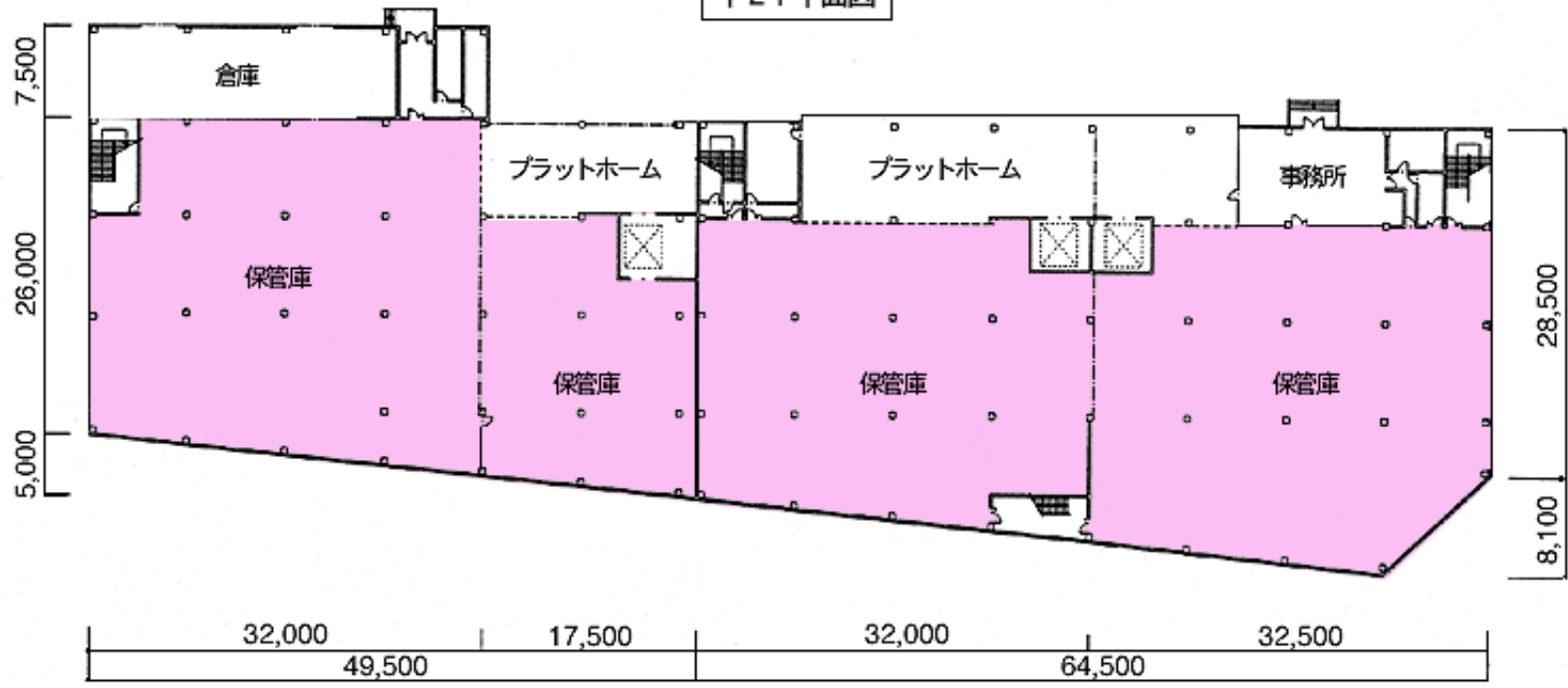
1F平面図
